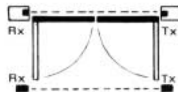
Fig. B CANCELLO A BATTENTE PORTAIL A BATTANTS SWING GATE FLÜGELTÖRE
